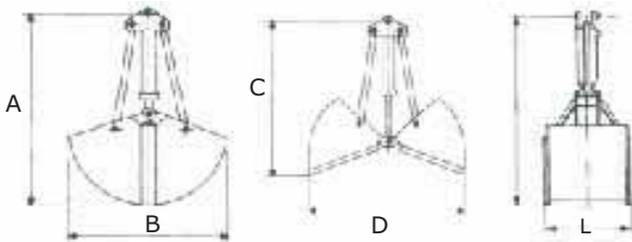
Croquis
