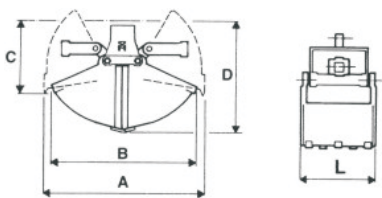
Croquis
