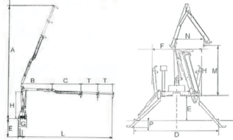
Dimensions
