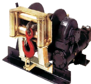
10,0 t treuil avec fenêtre à rouleaux
