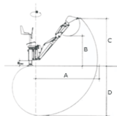
Croquis
