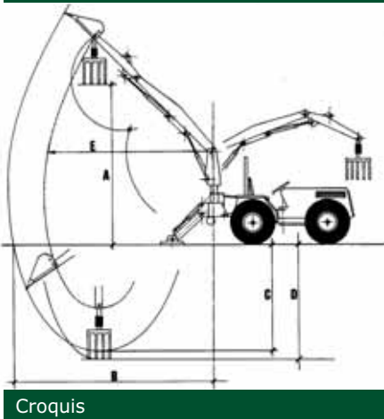
Grue CLN en terrassement
