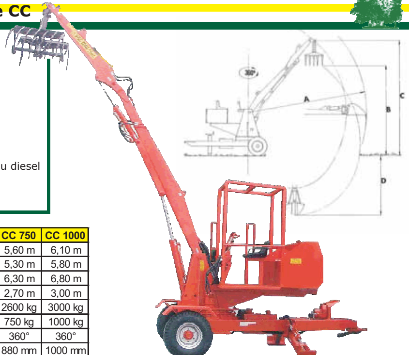
CC Chargeur sur essieu avec béquille hydraulique
