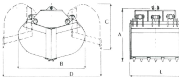
Croquis
