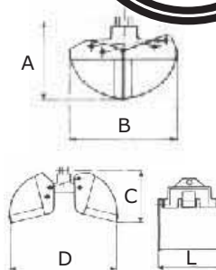
Croquis
