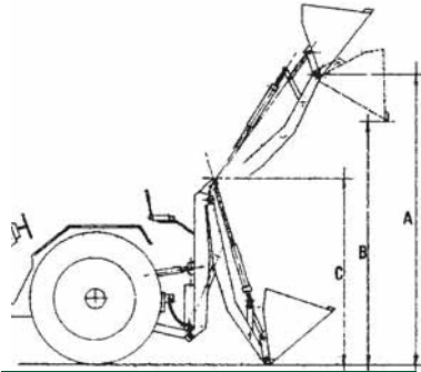
Croquis
